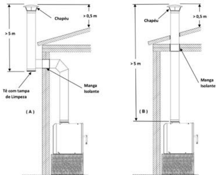
Figura 4. Diagrama da ligação do recuperador à chaminé
